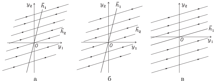
Рис. 2.12. Случай вырожденной матрицы.
