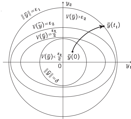
Рис. 2.4. К доказательству теоремы 2.4.1.
