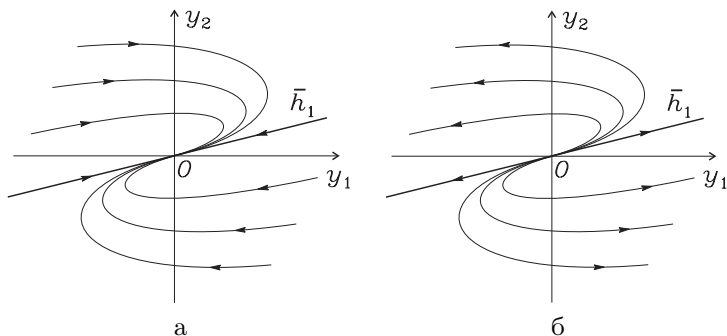
Рис. 2.8. Вырожденный узел: а – устойчивый, б – неустойчивый.
