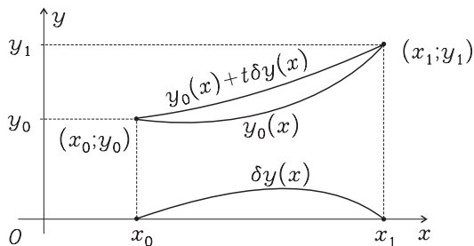
Рис. 5.2. К доказательству теоремы 5.2.1.
