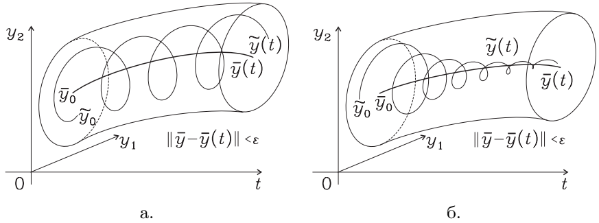
Рис. 2.2. К определениям устойчивости и асимптотической устойчивости решения \bar{y}(t) = \bar{y}(t; \bar{y}_0) :
