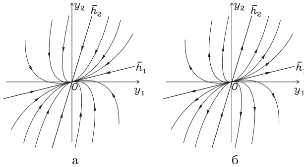
Рис. 2.6. Узел: а – устойчивый, б – неустойчивый.
