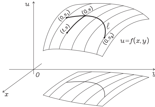
Рис. 4.2. К доказательству теоремы 4.2.4.
