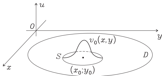
Рис. 5.4. К доказательству леммы 5.3.1.
