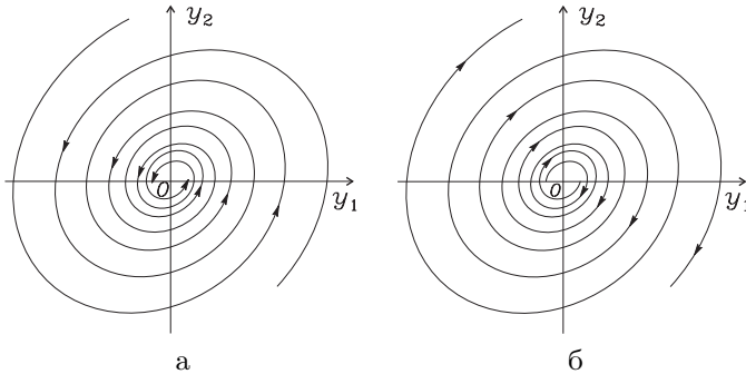
Рис. 2.10. Фокус: а – устойчивый, б – неустойчивый.
