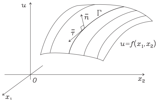
Рис. 4.1. К доказательству теоремы 4.2.3.
