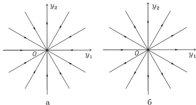
Рис. 2.7. Дикритический узел: а – устойчивый, б – неустойчивый.
