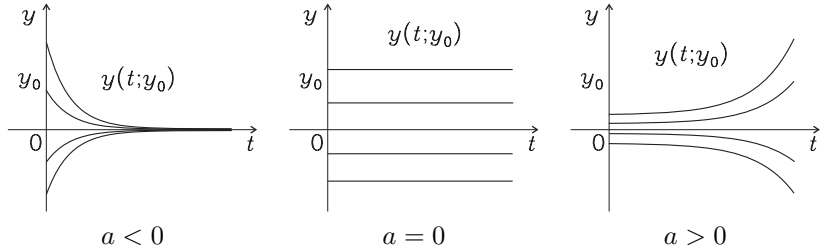
Рис. 2.1. К примеру 2.1.1: вид интегральных кривых решения задачи Коши y(t; y_0) = y_0 \exp\{at\} в зависимости от a .
