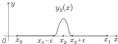
Рис. 5.1. К доказательству леммы 5.1.1.
