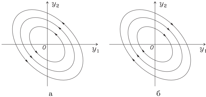
Рис. 2.11. Центр.
