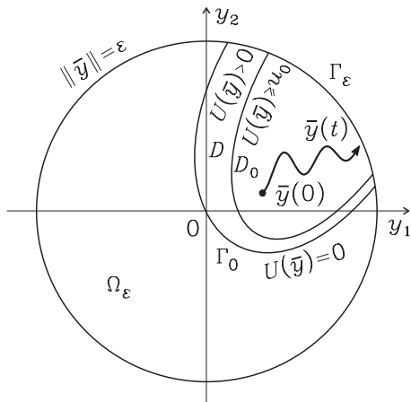
Рис. 2.5. К доказательству теоремы Четаева.
