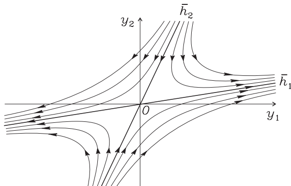
Рис. 2.9. Седло.
